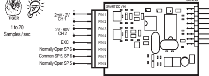
ISL1: Smart Dual LVDT. 50 Hz
